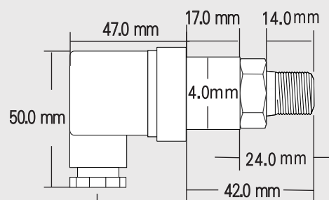
Connector: DIN 43650
