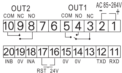
● CR6 (96x48mm)
